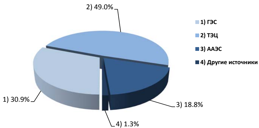
Производство электроэнергии по электростанциям, январь - июнь 2021г.
