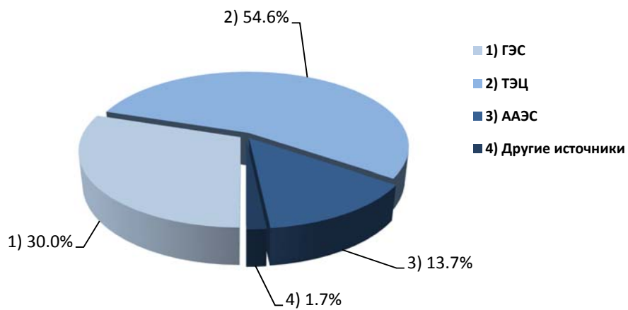
Производство электроэнергии по электростанциям, январь - август 2021г.
