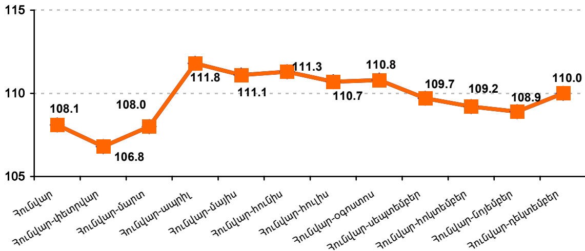
Մանրածախ առևտրի ֆիզիկական ծավալի ինդեքսները 1 2007թ. հունվար-դեկտեմբերին 2006թ. համապատասխան ժամանակաշրջանի նկատմամբ (համադրելի գներով, %)
