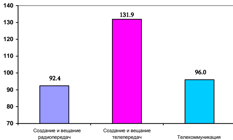
Индексы физических объемов создания, вещания телерадиопередач и телекоммуникационной связи за IV квартал 2019г. по сравнению с соответствующим периодом предыдущего года
